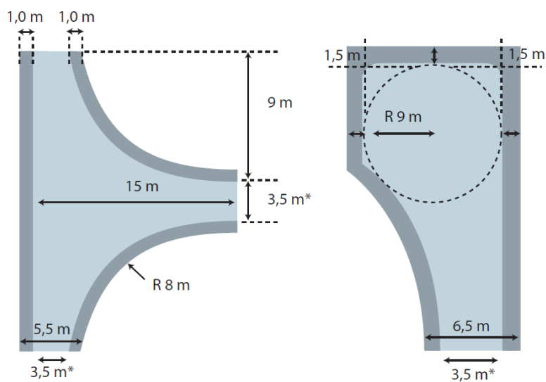
Figur 3 Exempel på vändplatser
